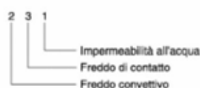
Classificazione delle prestazioni di resistenza al freddo dei guanti
